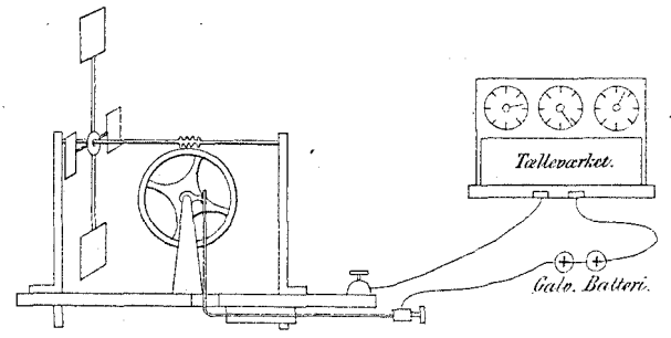
Anemometret. Fig. 10.
